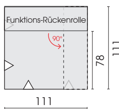
Element tief mit Funktionsrücken, rechts 11T
