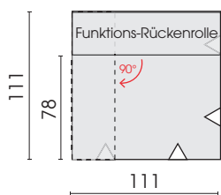
Element tief mit Funktionsrücken, links 12T
