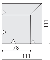
Eckelement tief, rechts 71T
