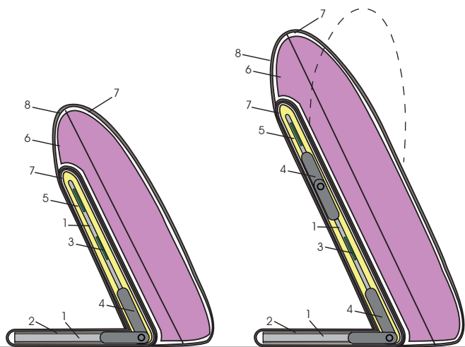
Modell 1070 / TYP 611/612
